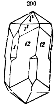
Pyrrargyrite.
